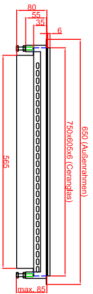
Variante "B" Ausschnitt in Abdeckung flächenbündiger Einbau 758mm x 613mm
