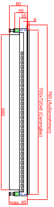
Variante "B" Ausschnitt in Abdeckung flächenbündiger Einbau 708mm x 728mm
