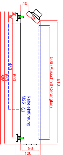
Seitenansicht
