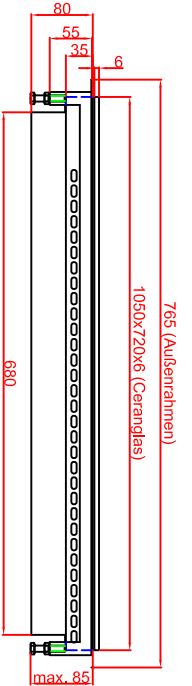
Variante "B" Ausschnitt in Abdeckung flächenbündiger Einbau 1058mm x 728mm
