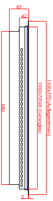
Variante "A" Ausschnitt in Abdeckung Einbau mit Auflagerahmen 1080mm x 750mm
