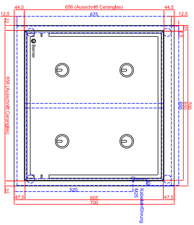
Draufsicht
