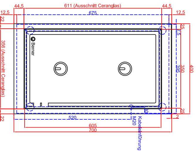
Draufsicht
