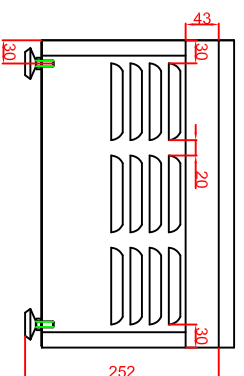
Rückansicht
