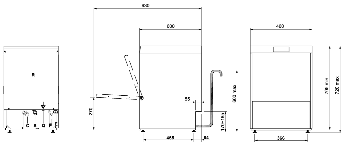
Gläserpülmaschine Korb 400 x 400 mm - Serie UG415
