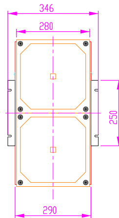
Generatoransicht generator view
