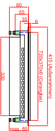
Variante "B" Ausschnitt in Abdeckung flächenbündiger Einbau 728mm x 378mm
