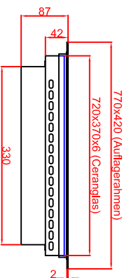
Variante "A" Ausschnitt in Abdeckung Einbau mit Auflagerahmen 750mm x 400mm
