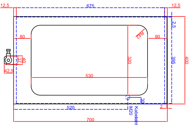
Draufsicht
