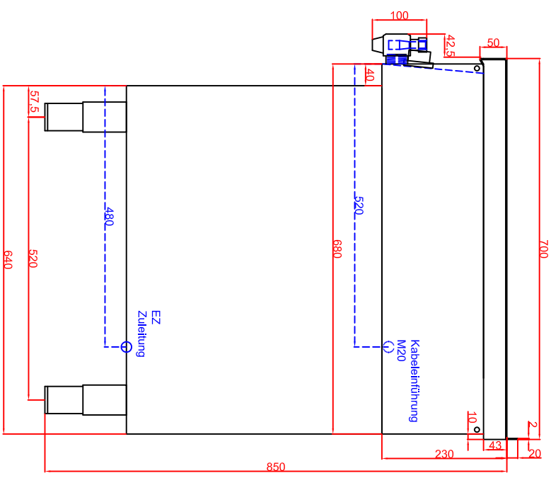
Seitenansicht
