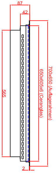
Variant "A" Ausschnitt in Abdeckung Einbau mit Auflagerahmen 680mm x 630mm
