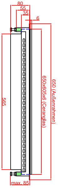
Variant "B" Ausschnitt in Abdeckung flächenbündiger Einbau 658mm x 613mm
