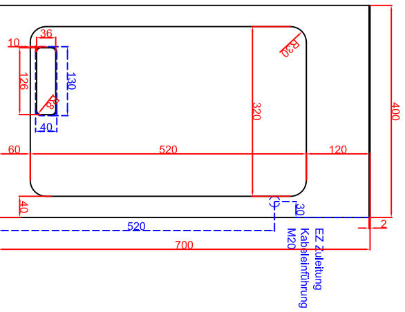
Draufsicht
