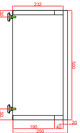
Rückansicht
