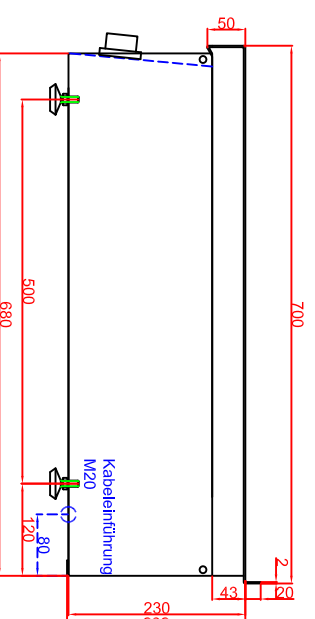
Seitenansicht
