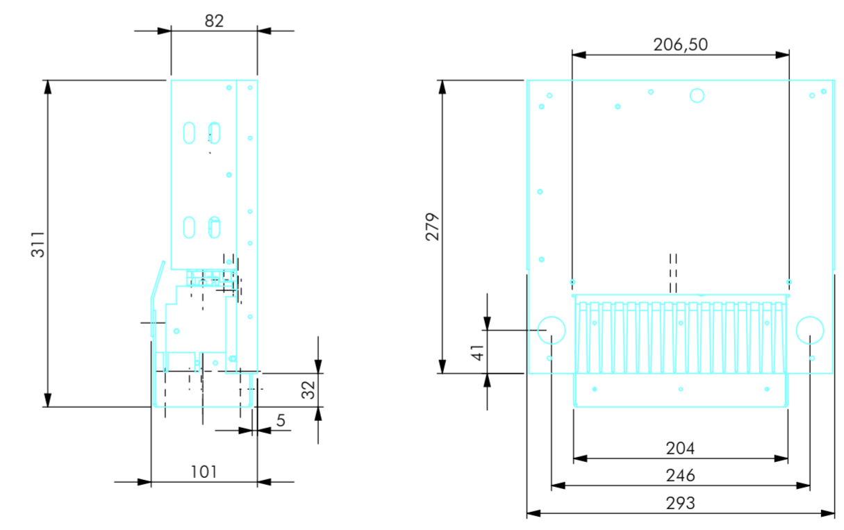
Generatoransicht generator view
