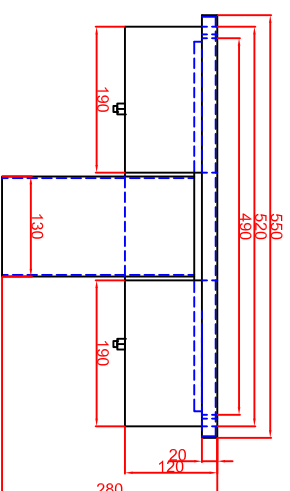
Seitenansicht
