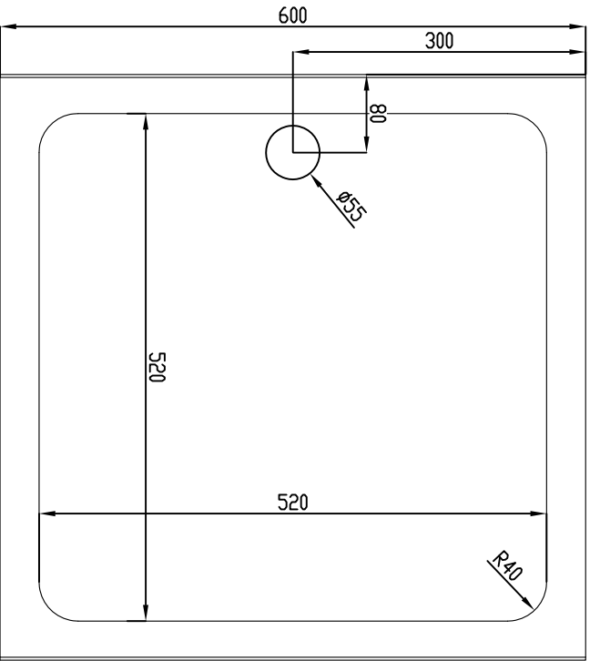
Draufsicht
