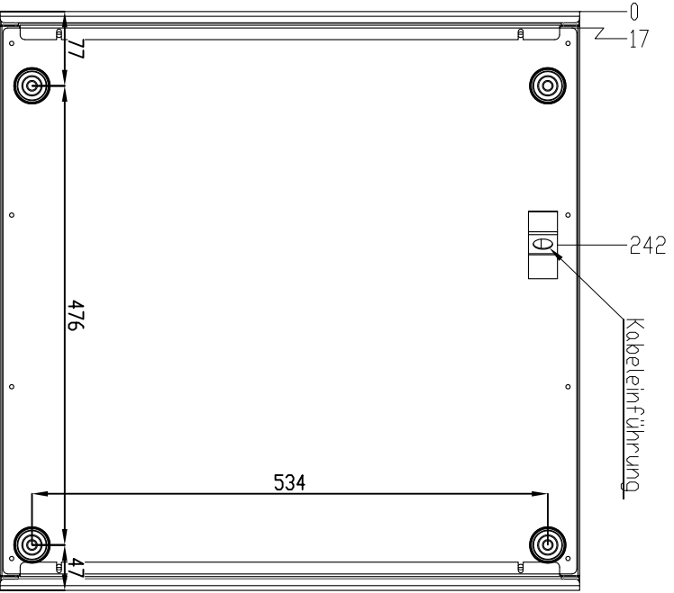
Unteransicht
