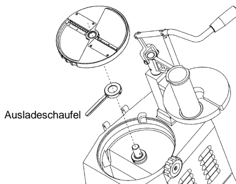
Demontage und Montage der Ausladeschaufel
