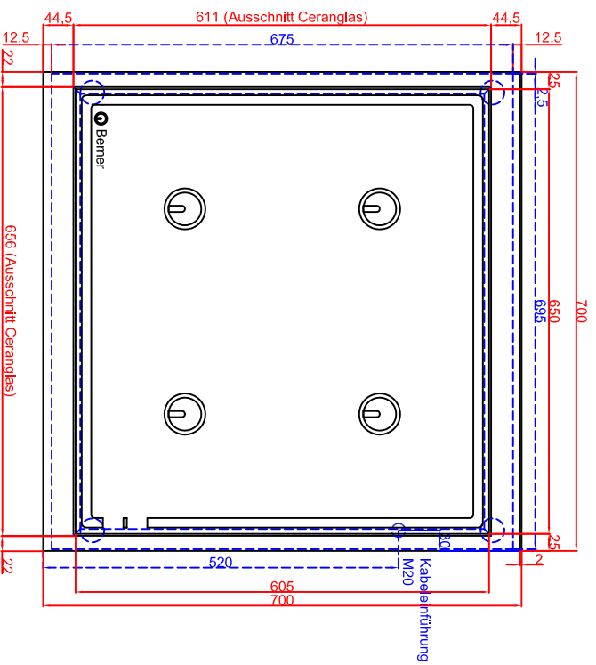
Draufsicht
