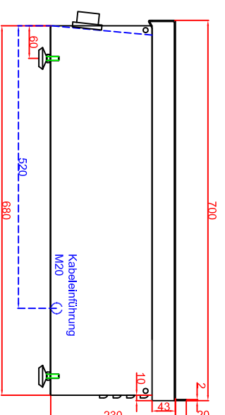
Seitenansicht
