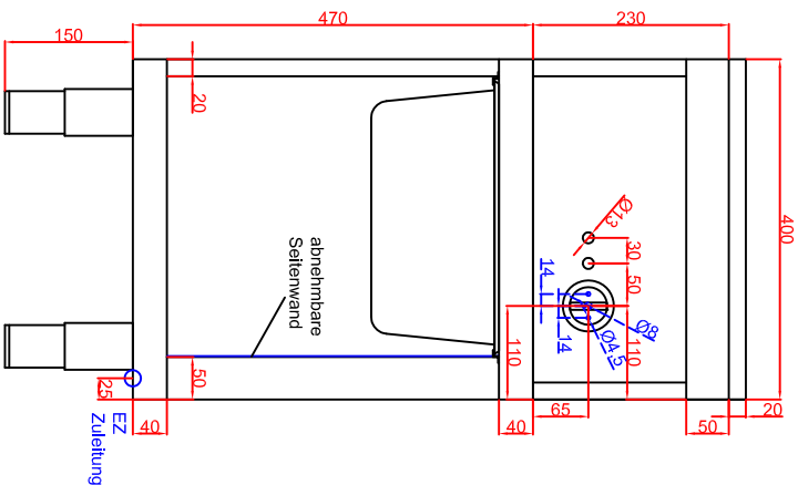
Frontansicht
