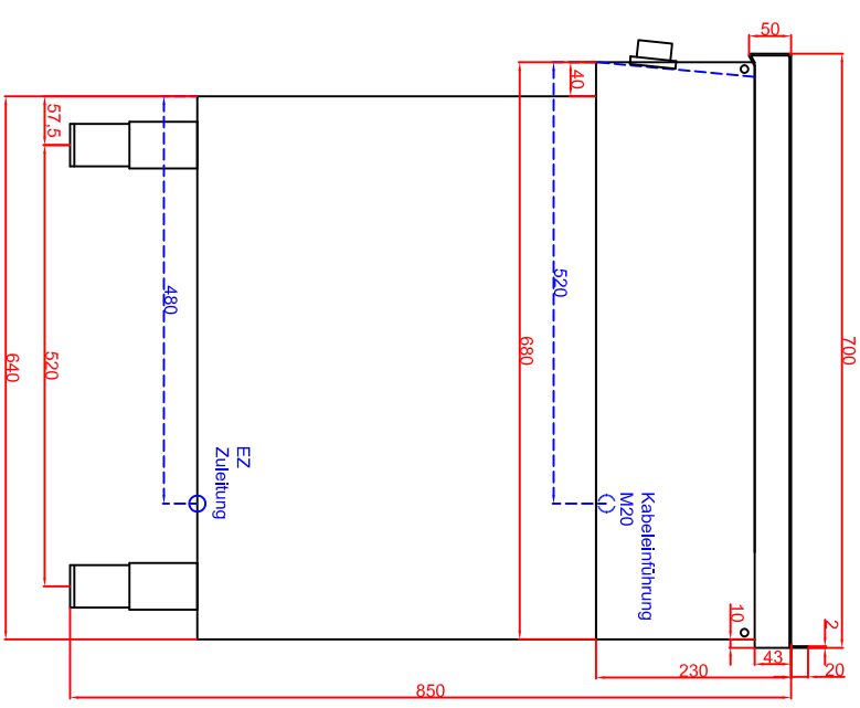
Seitenansicht
