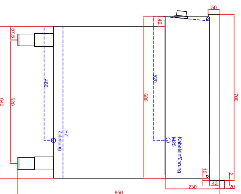
Seitenansicht
