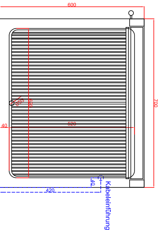
Draufsicht
