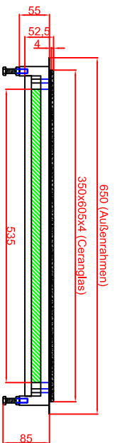
Ausschnitt in Abdeckung flächenbündiger Einbau 356mm x 611mm
