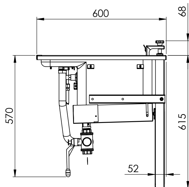
Seitenansicht / Side view
