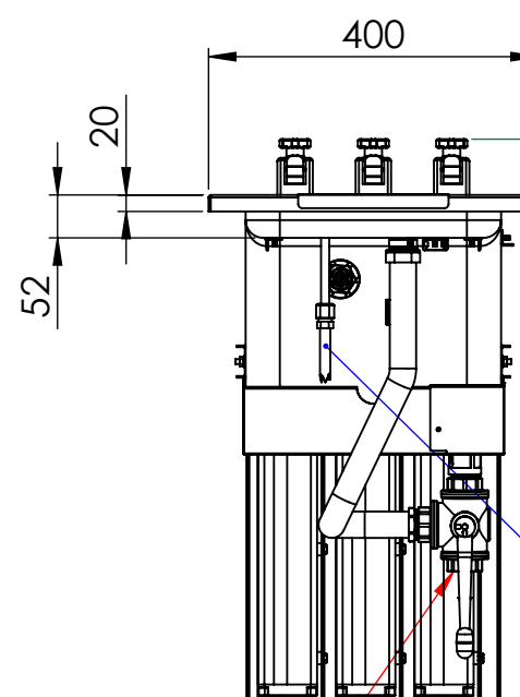
Vorderansicht / Front view
