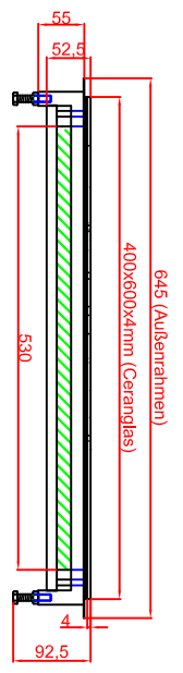
Variante "B" Ausschnitt in Abdeckung flächenbündiger Einbau 406mm x 606mm
