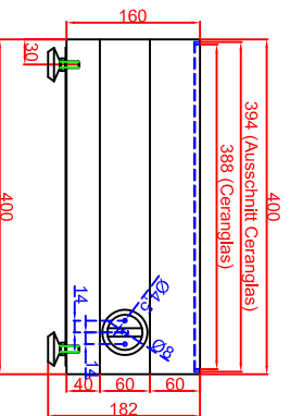
Frontansicht
