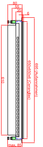
Variante "B" Ausschnitt in Abdeckung flächenbündiger Einbau 658mm x 658mm
