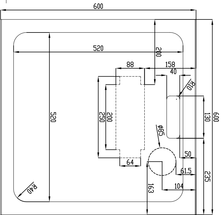
Draufsicht
