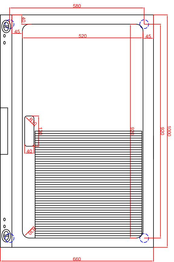
Draufsicht
