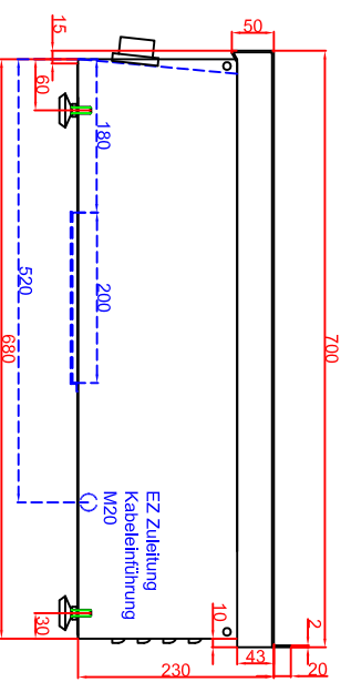
Seitenansicht
