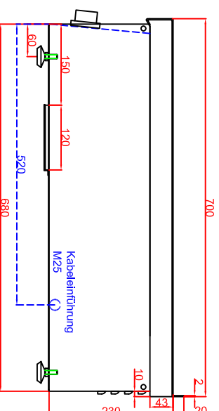
Seitenansicht
