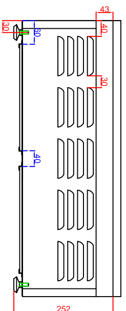
Rückansicht
