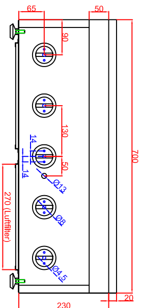
Frontansicht
