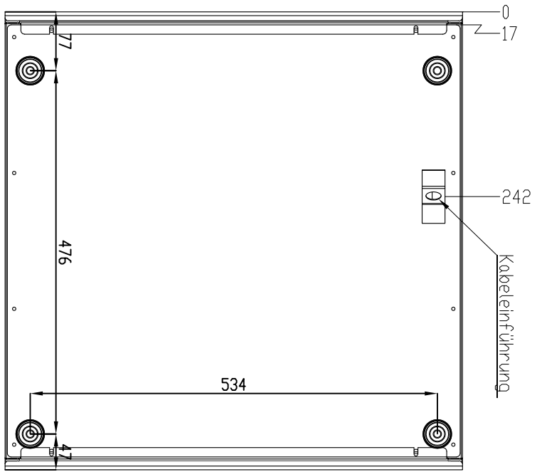
Unteransicht
