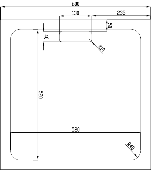
Draufsicht
