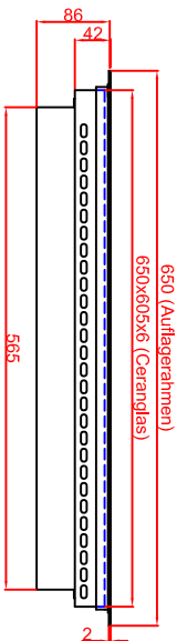
Variante "A" Ausschnitt in Abdeckung Einbau mit Auflagerahmen 680mm x 630mm
