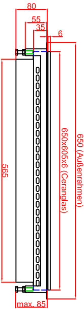
Variante "B" Ausschnitt in Abdeckung flächenbündiger Einbau 658mm x 613mm
