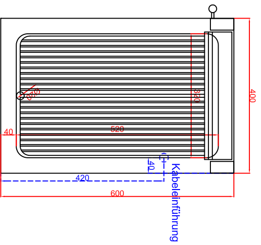
Draufsicht
