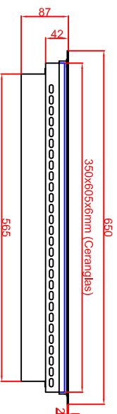
Variante "A" Ausschnitt in Abdeckung Einbau mit Auflagerahmen 380mm x 630mm
