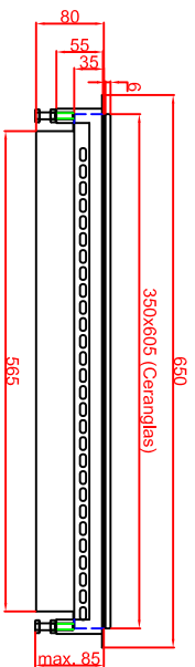
Variante "B" Ausschnitt in Abdeckung flächenbündiger Einbau 358mm x 613mm
