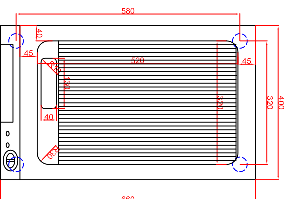
Draufsicht
