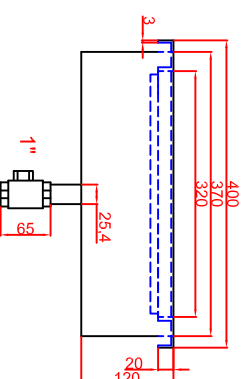
Frontansicht
