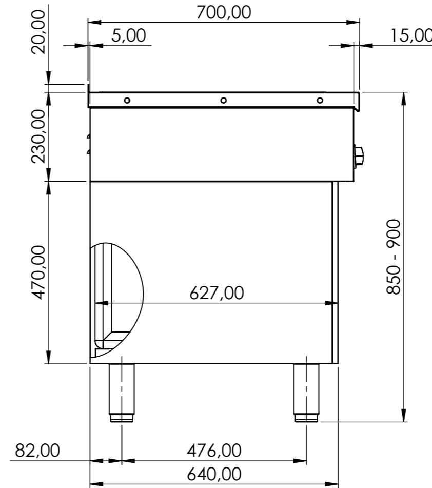
Seitenansicht / side view
