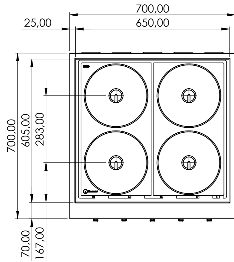
Draufsicht / top view
